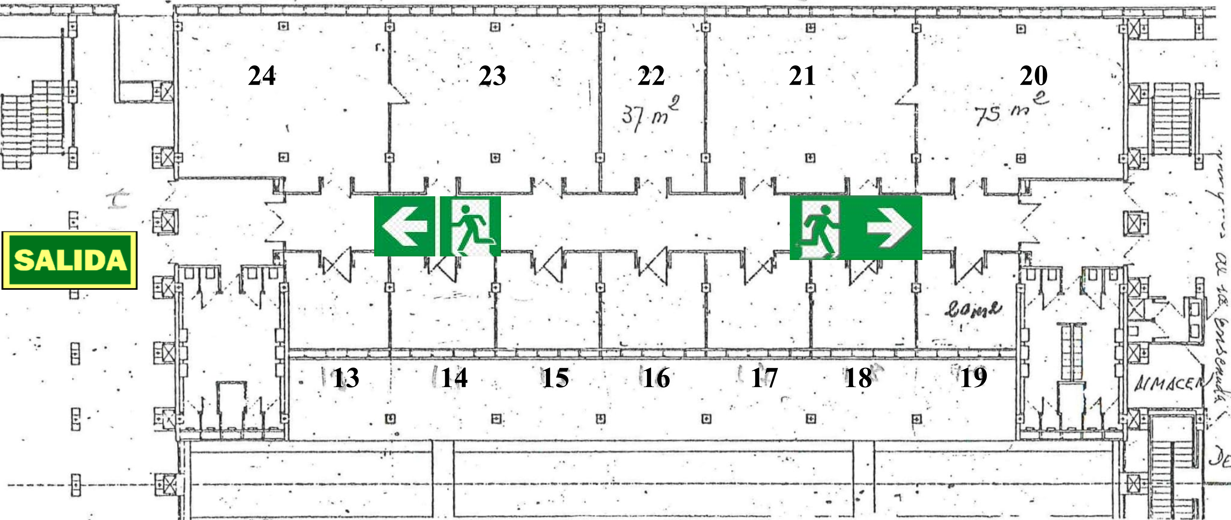
PLANTA BAIXA
